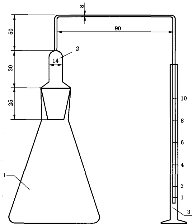
图中： 1——100 mL 锥形瓶，用于发生砷化氢； 2——连接管，用于捕集硫化氢； 3——10 mL 量筒，吸收砷化氢用。
